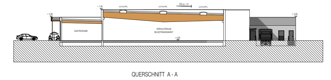
Schnitt (südliches Gebäude) | M 1:500
