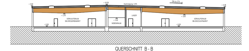
Schnitt (südliches Gebäude) | M 1:500
